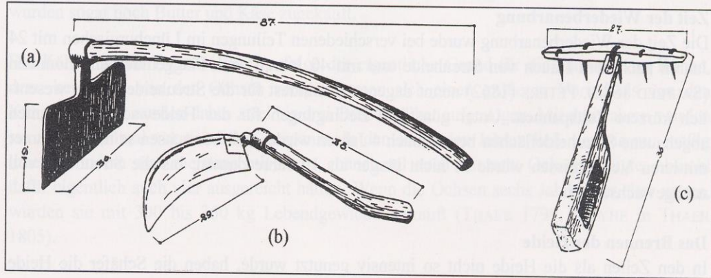
Abb. 14: Geräte zum Heide- und Plaggenhieb: Twicke (a), Heidlinne (b) und Heideharke (c) nach BOMANN (1933/1992)
